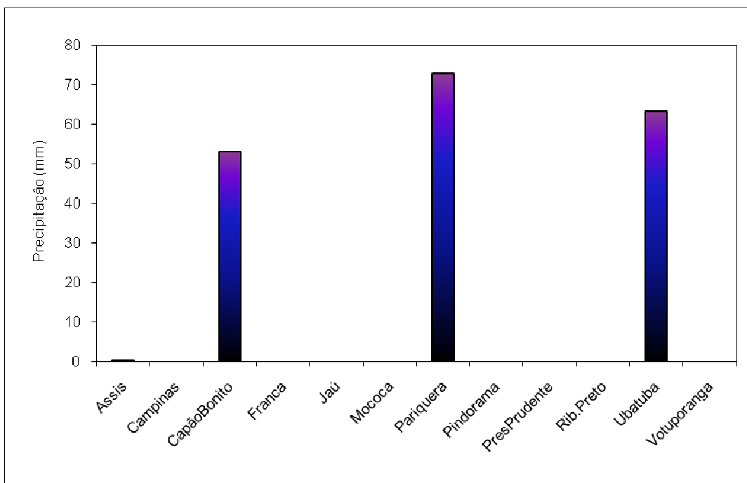
Figura 3 – Volume total de precipitação acumulada no mês de Agosto para localidades do estado de São Paulo. Fonte: Ciiagro
