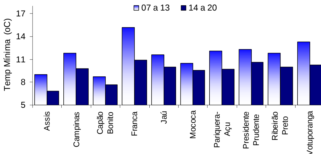
Figura 2 – Temperatura mínima, média do período anterior comparada com as medias do período atual para localidades do estado de São Paulo.
