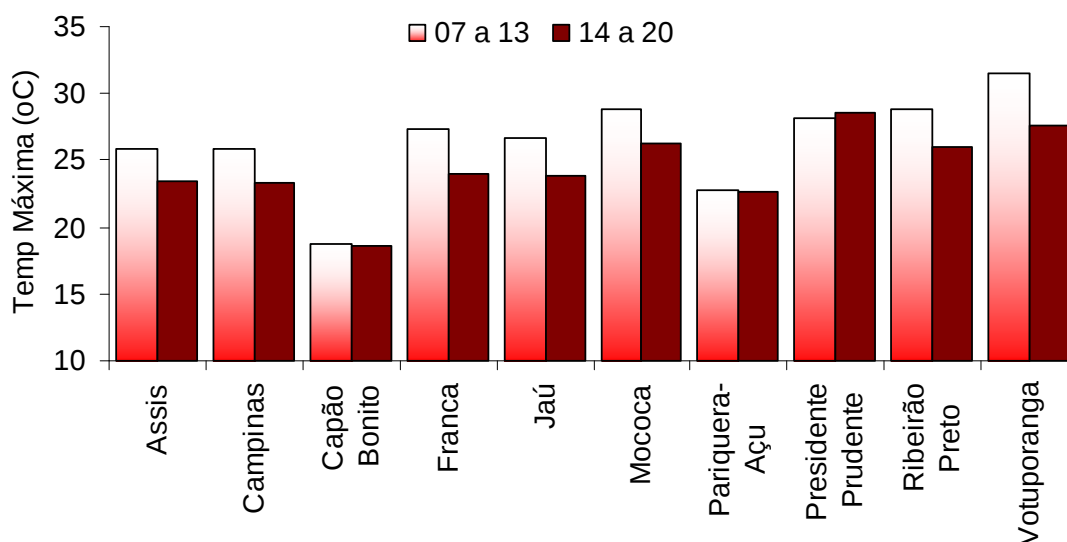
Figura 1 – Temperatura máxima, média do período anterior comparada com as medias do período atual para localidades do estado de São Paulo.
