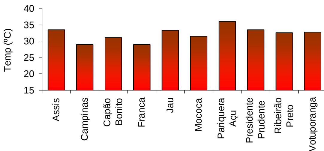
Figura 1 – Temperatura máxima, média do período de 30/01 a 05/02 para localidades do estado de São Paulo.
