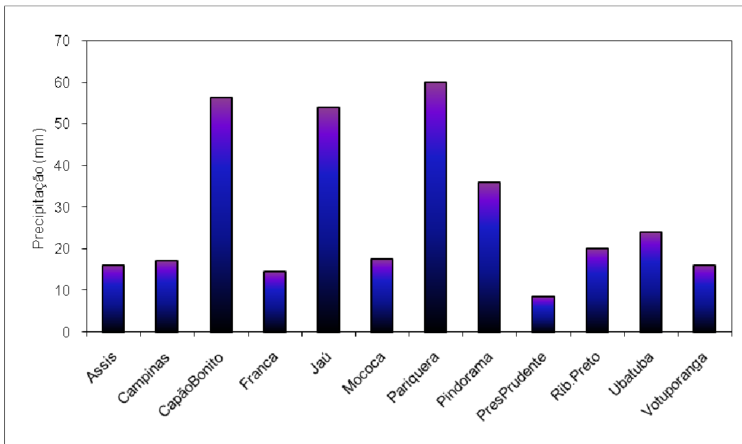
Figura 3 – Volume total de precipitação acumulada no período analisado (30/01 a 05/02/2010), para localidades do estado de São Paulo. Fonte: Ciiagro
