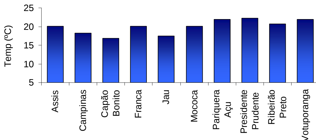
Figura 2 – Temperatura mínima, média do período de 30/01 a 05/02 para localidades do estado de São Paulo.
