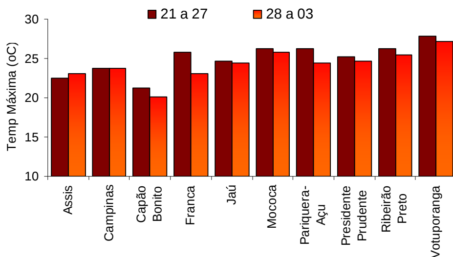
Figura 1 – Temperatura máxima, média do período de 21 a 27/05 comparadas com o período atual de 28/05 a 03/06, para localidades do estado de São Paulo.
