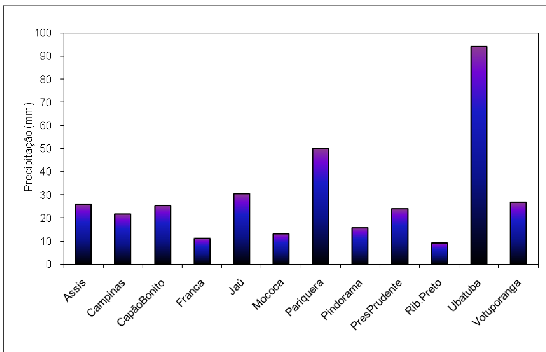
Figura 3 – Volume total de precipitação acumulada no período analisado (04 a 10/06/2010), para localidades do estado de São Paulo. Fonte: Ciiagro
