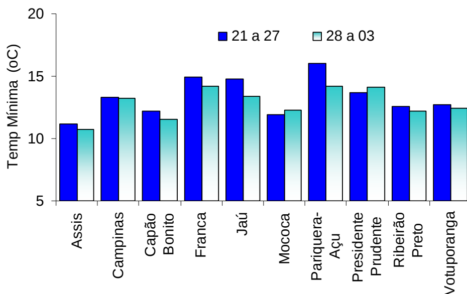
Figura 2 – Temperatura mínima, média do período de 21 a 27/05 comparadas com o período atual de 28/05 a 03/06, para localidades do estado de São Paulo.
